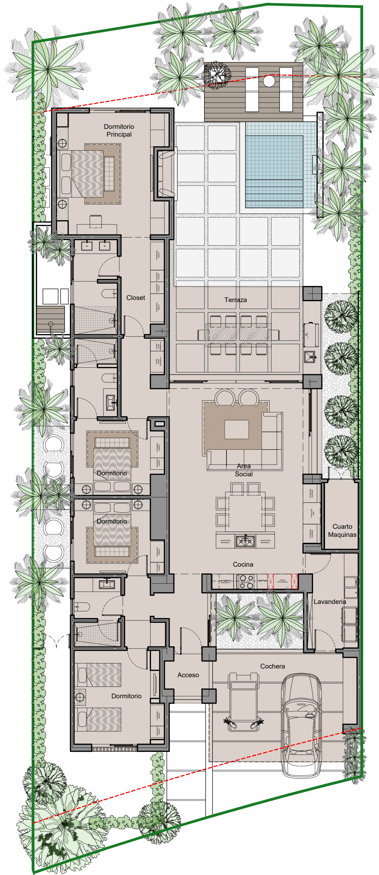
Sueños del Mar Casa D - Decor/+ nivel 0+0.00m N1 Habitable: 259.40m2 N1 Terraza Abierta: 29.56m2 N1 Piscina: 11.20m2 construccion permitida en lotes 4-10-11-13-14
